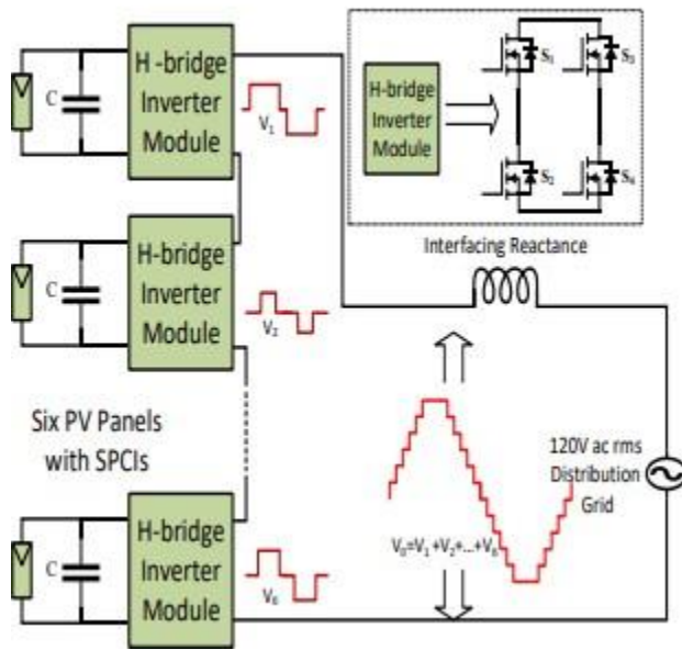
Fig.1. Block diagram.
