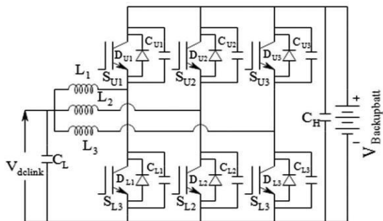
Fig.3.1. BIDC circuit.
